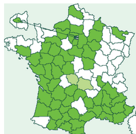
Fig. n° 3: Carte de répartition d' Eublemma purpurina sur Lepinet incluant la donnée.
