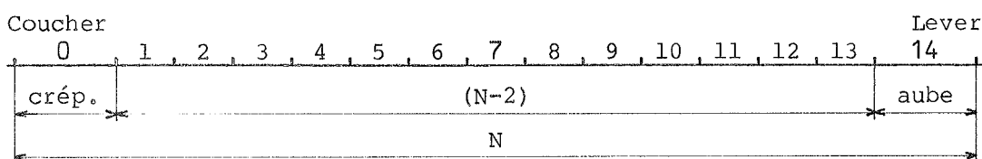
Fig. 2. - Numérotation des périodes (pM).
