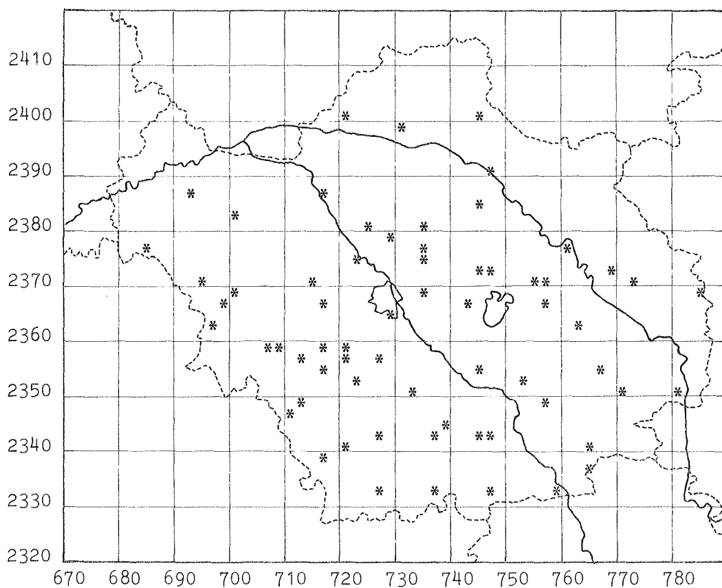
Fig. 1. - Carte de répartition des stations de Noctuidae. Grille Lambert II étendu - *2 km.
